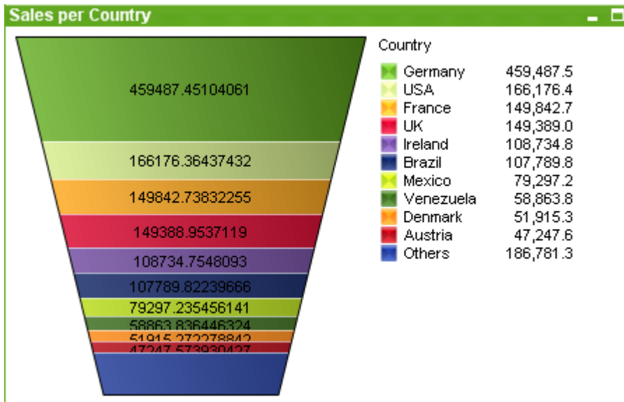
Pivot table
